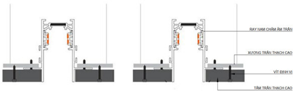
HÌNH MINH HỌA THI CÔNG LẮP ĐẶT RAY TRẦN
